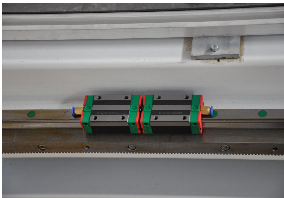
Hiwin - направляющая и блок скольжения
