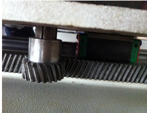
Косозубая рейка и шестерня
